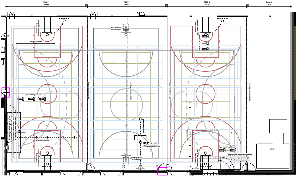
belijningsplan
